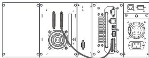
Рисунок 2. Кабельные соединения SCSI для одного устройства
