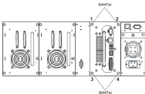
Рисунок 1. Установка SNC в библиотеку Dell PowerVault 132T.
