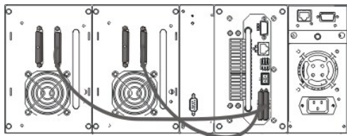
Рисунок 3. Кабельные соединения SCSI для двух устройств
